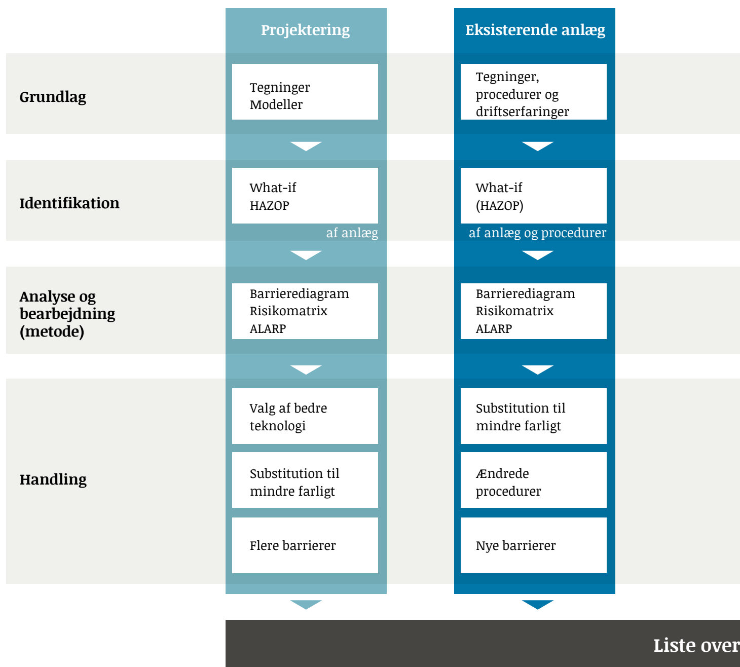
Figur 17 Figuren viser, hvordan der kan udføres risikovurdering i projekteringsfasen, ved undersøgelse af eksisterende anlæg og ved daglige observationer. Det bærende element for virksomheder med komplicerede processer er en opdateret liste over barrierer (sikkerhedsforanstaltninger).
