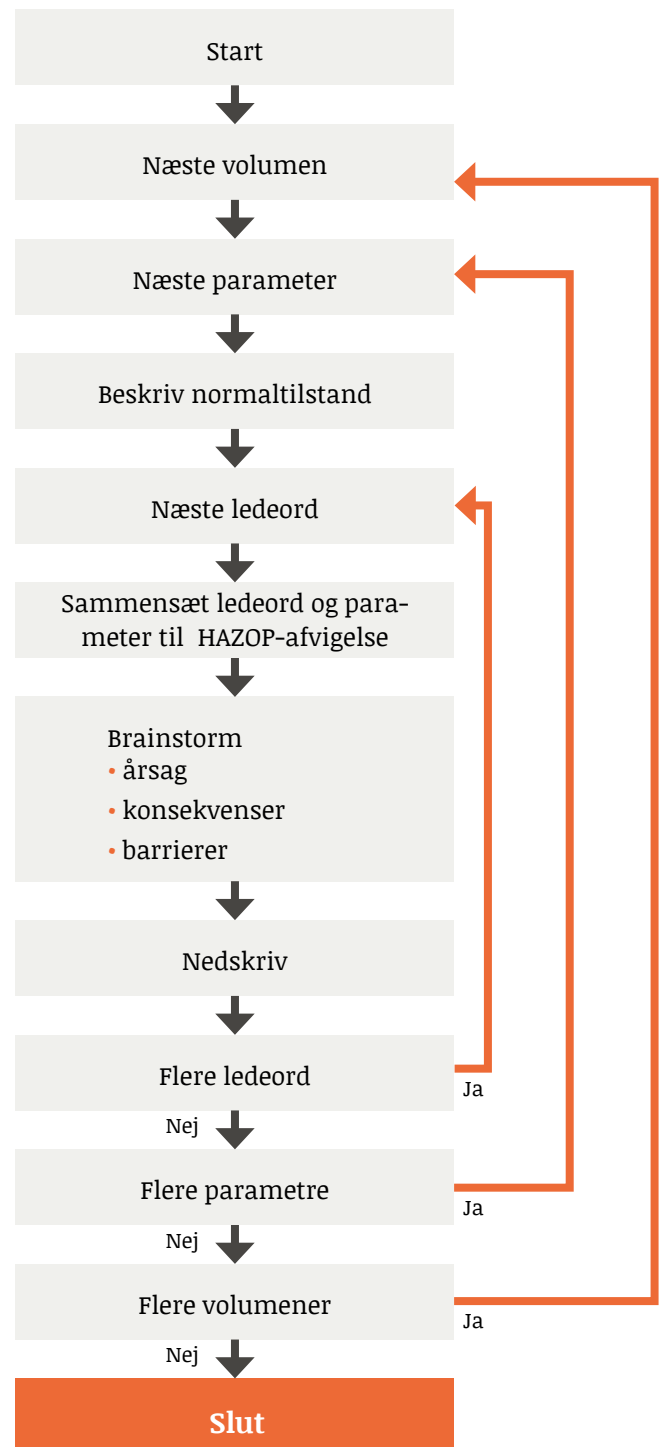
Figur 11 Skematisk beskrivelse af HAZOP-fremgangsmåden.
